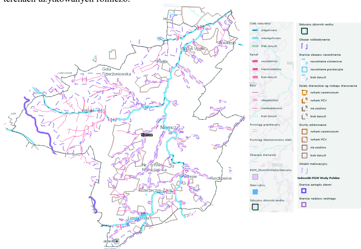
Rysunek 4 Obszary gruntów zmeliorowanych na tle Gminy Niemcza, źródło: opracowanie własne
