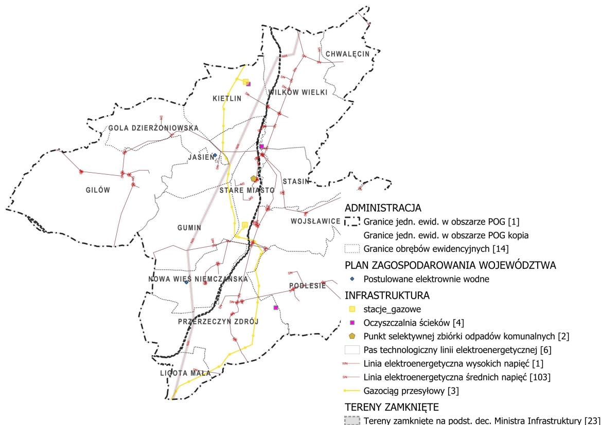
Rysunek 9 Infrastruktura techniczna , źródło: opracowanie własne
