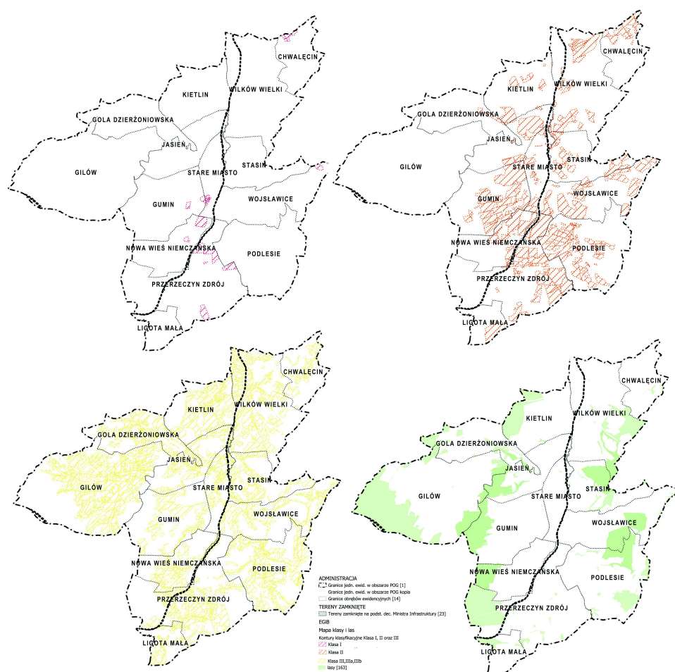
Rysunek 8 Grunty rolne stanowiące użytki rolne klasy I-III oraz grunty leśne na terenie gminy Niemcza, źródło: opracowanie własne
