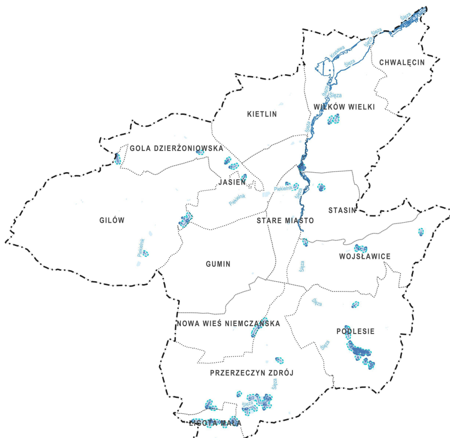
Rysunek 3 Obszary szczególnego zagrożenia powodzią, wały przeciwpowodziowe oraz pasy od stopy wały w Gminie Niemcza, źródło: opracowanie własne
