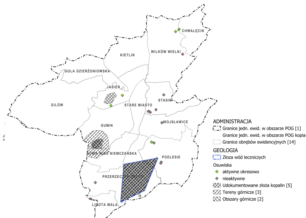
Rysunek 5 Mapa z lokalizacją złóż leczniczych, osuwisk, udokumentowanych złóż kopalin wraz z terenami górniczymi oraz obszarami górniczymi na terenie Gminy Niemcza, źródło: opracowanie własne
