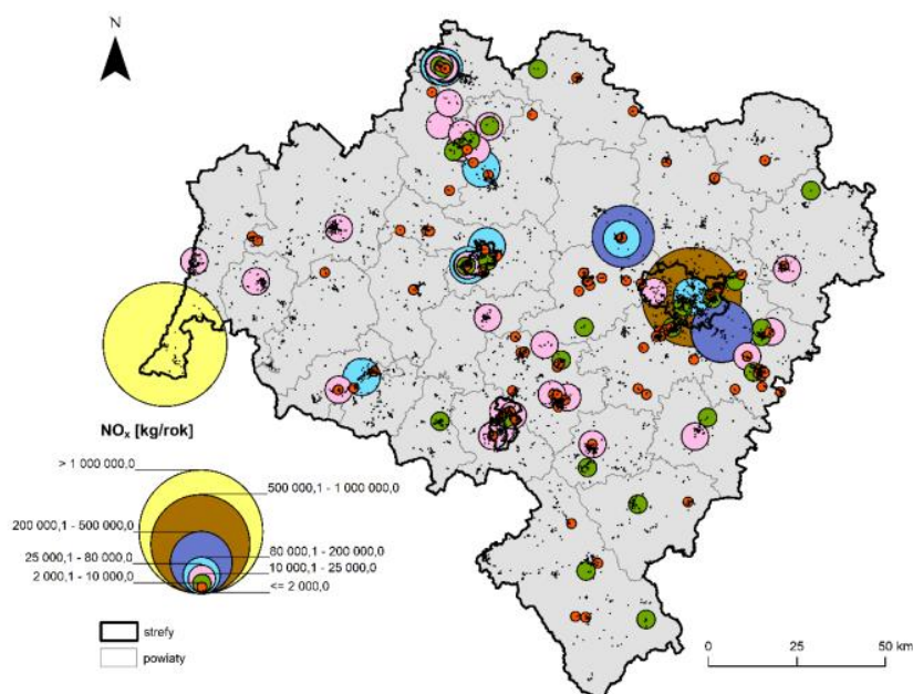
Rysunek 1-53 Rozmieszczenie oraz ładunki emisji punktowej NO x w województwie dolnośląskim w 2021 r.
