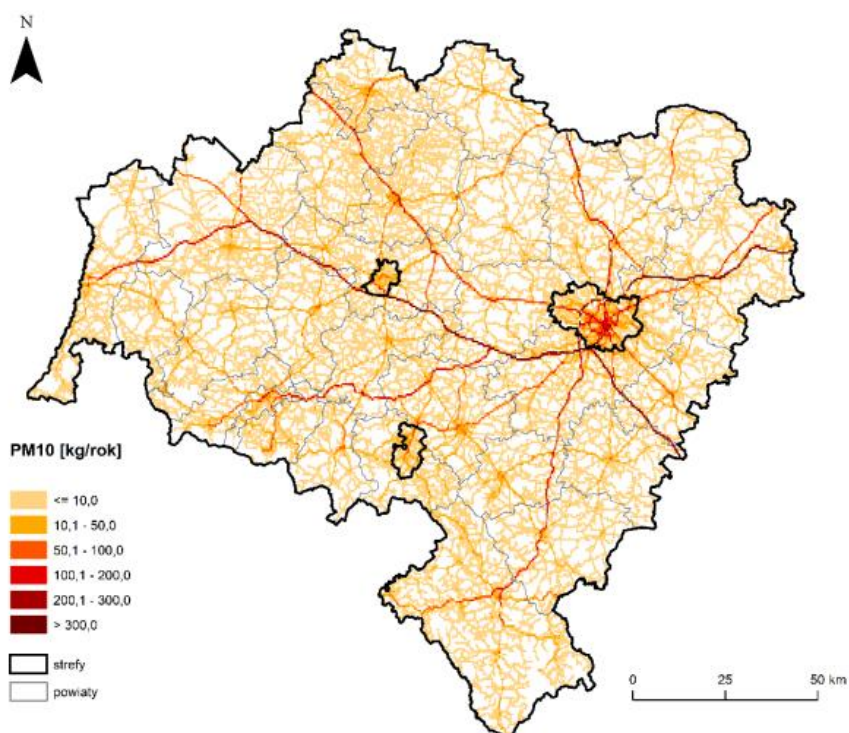
Rysunek 1-56 Rozmieszczenie oraz ładunki emisji liniowej pyłu zawieszony PM10 w województwie dolnośląskim w 2021 r.
