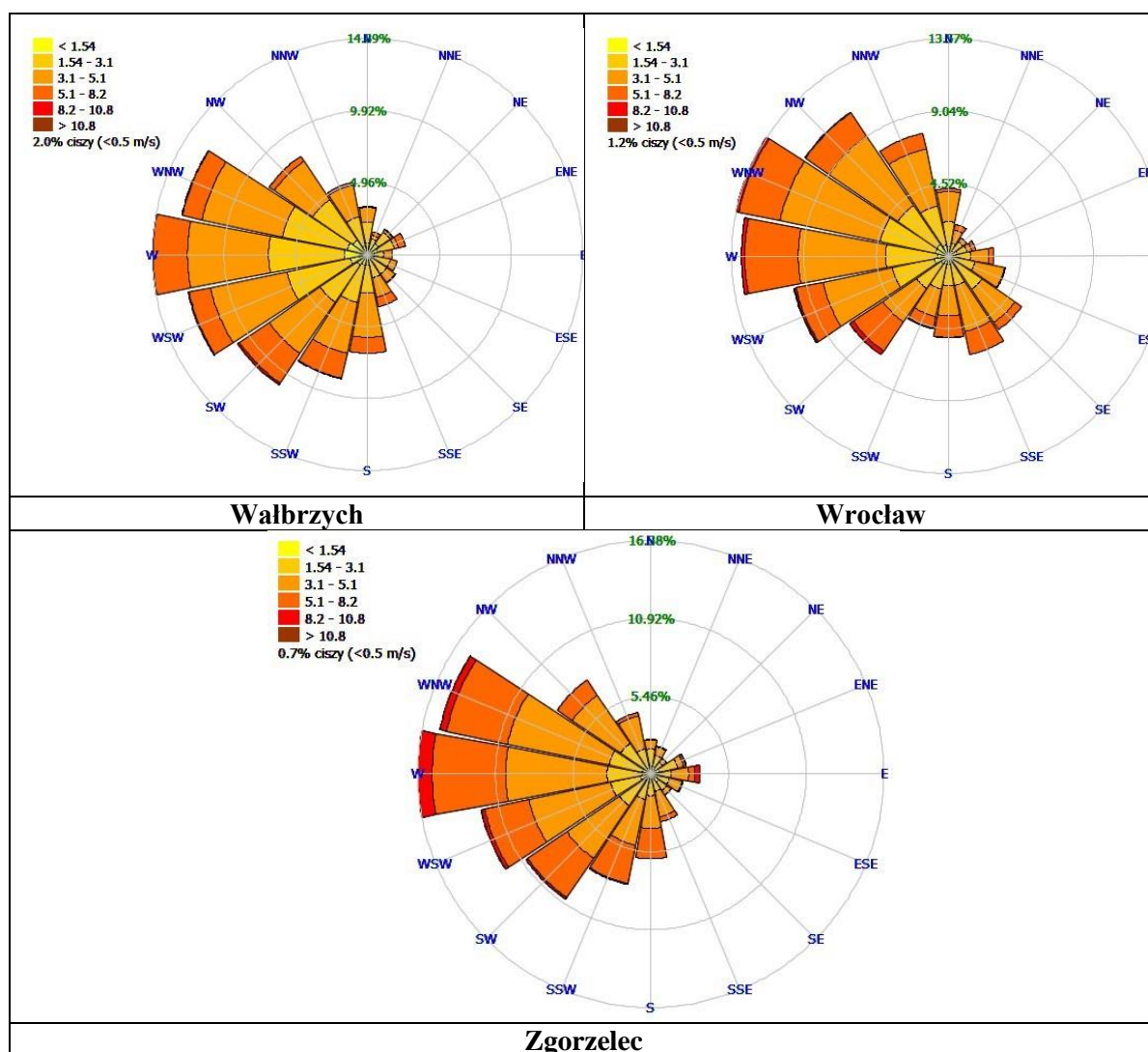
Rysunek 1-22 Rozkład kierunków i prędkości wiatru dla miejscowości w województwie dolnośląskim w 2021 r.
