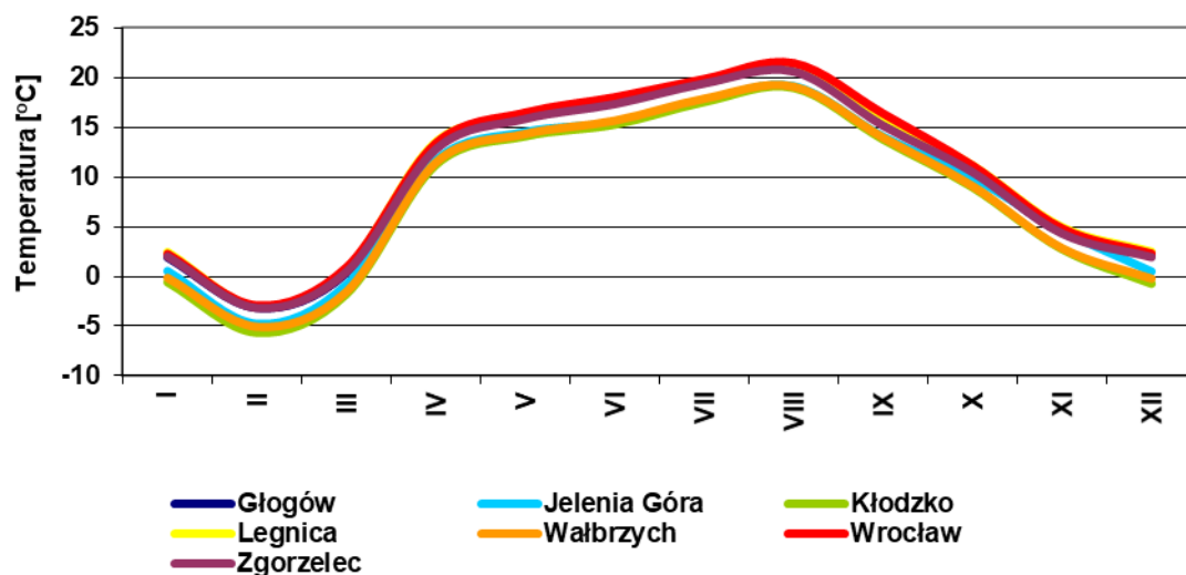
Rysunek 1-24 Przebiegi średnich miesięcznych temperatur powietrza wyznaczone przez model WRF/CALMET w wybranych miejscowościach województwa dolnośląskiego w 2018 r.
