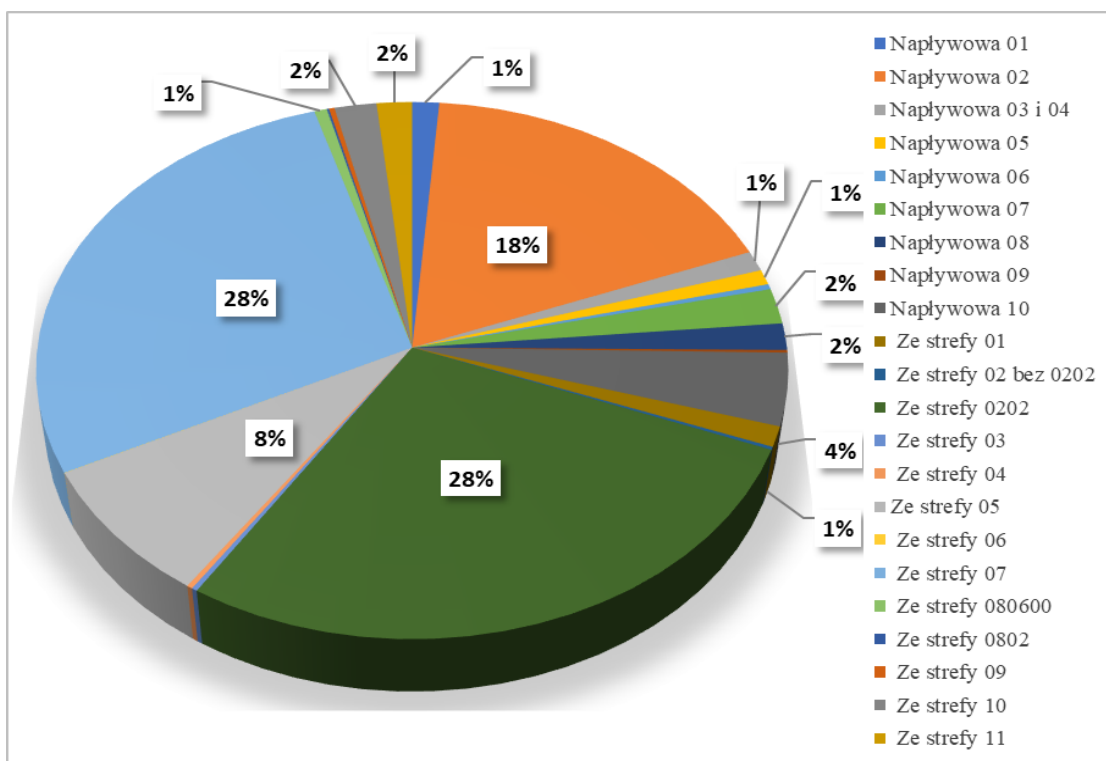
Rysunek 1-59 Udział % typów emisji pyłu zawieszonego PM10 dla strefy dolnośląskiej, w 2018 r.
